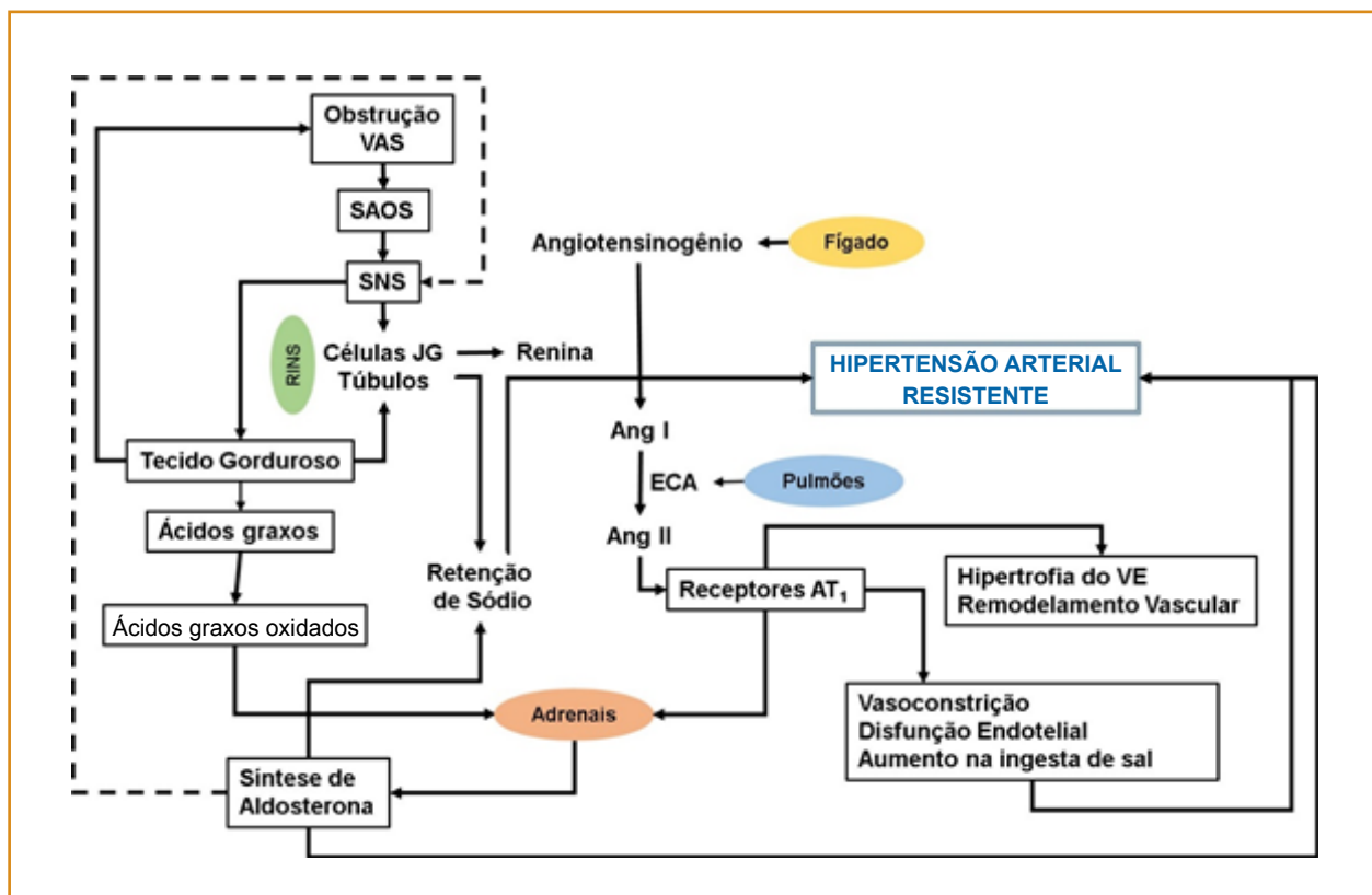
Figura 16.4. Sistemas biomoleculares mediando o desequilíbrio entre a síntese aumentada de aldosterona, a retenção de sódio, a AOS, a atividade aumentada do SRAA (receptores AT 1 e AT 2 ) e a cardiopatia hipertensiva e resistência vascular total aumentada, induzidas principalmente pela expansão do volume plasmático (retenção de sal e excesso de aldosterona) e pela hiperatividade simpática.
